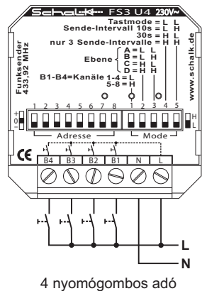
FS3 U4 adó
