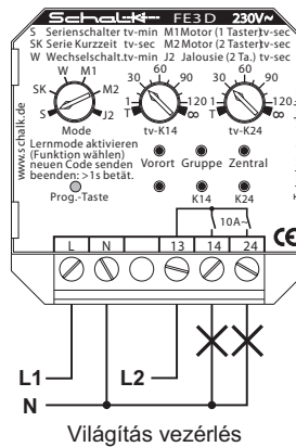
FE3 D(V) vevő 2 relével (2 Záró [10A] kapcsolással)
