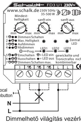
FD3 U1 univerzális dimmer 500W
