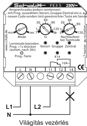
FE3 S(V) vevő1 relével (1 Váltó [10A] kapcsolással)
