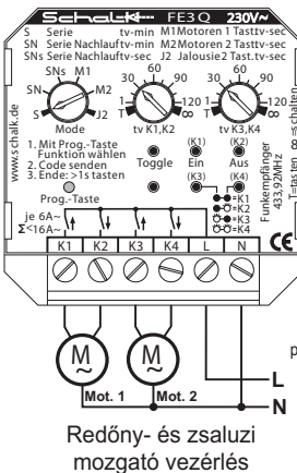
FE3 Q vevő 4 relével (4 Záró [6A] kapcsolással)
