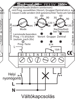
FE3 S(V) vevő1 relével (1 Váltó [10A] kapcsolással)
