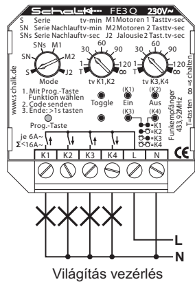
FE3 Q vevő 4 relével (4 Záró [6A] kapcsolással)
