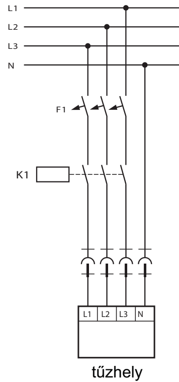
3 fázisú fogyasztó időzített kapcsolása ZS U2-vel.
