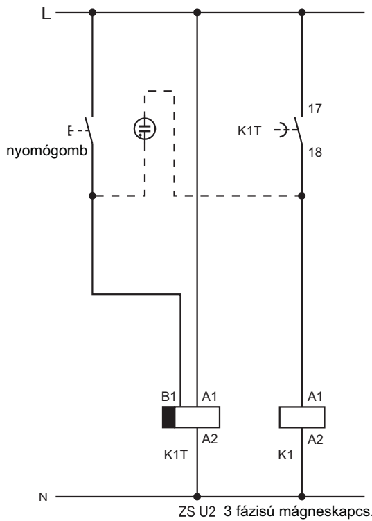
3 fázisú fogyasztó időzített kapcsolása ZS U2-vel.
