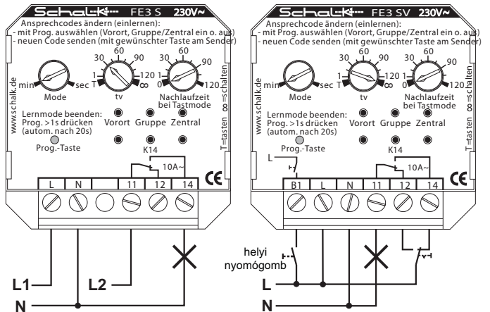
FE3 S(V) vevő 1 relével
