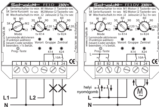
FE3 D(V) vevő 2 relével
