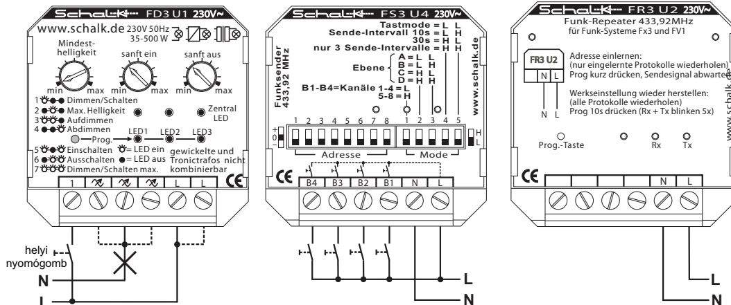
FD3 U1 univerzális dimmer FS3 U4 kötődobozba szerelhető adó FR3 U2 ismétlő (repeater)
